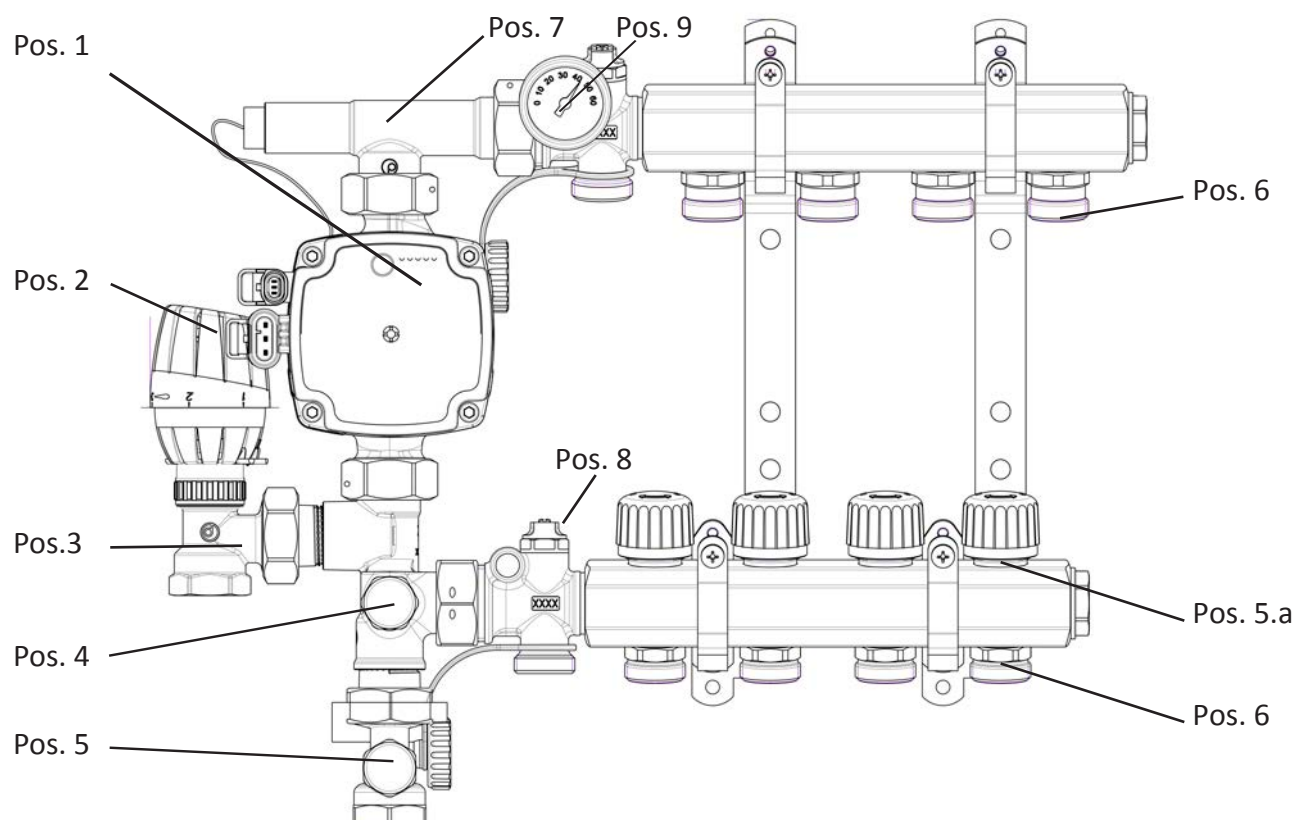
KVIKSHUNT - ALSK20UPM3-XX - 2 TIL 12 KREDSE (RESERVEDELSLISTE)
