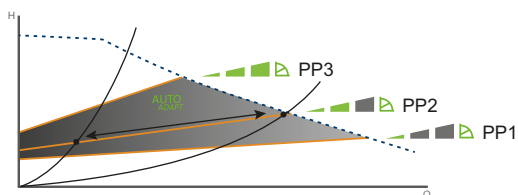
Fig. 22 Tre proportionaltrykkurve/-indstillinger
